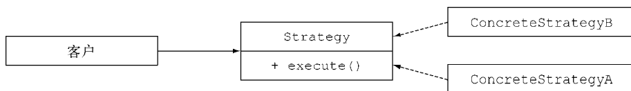
图8-1 策略模式
